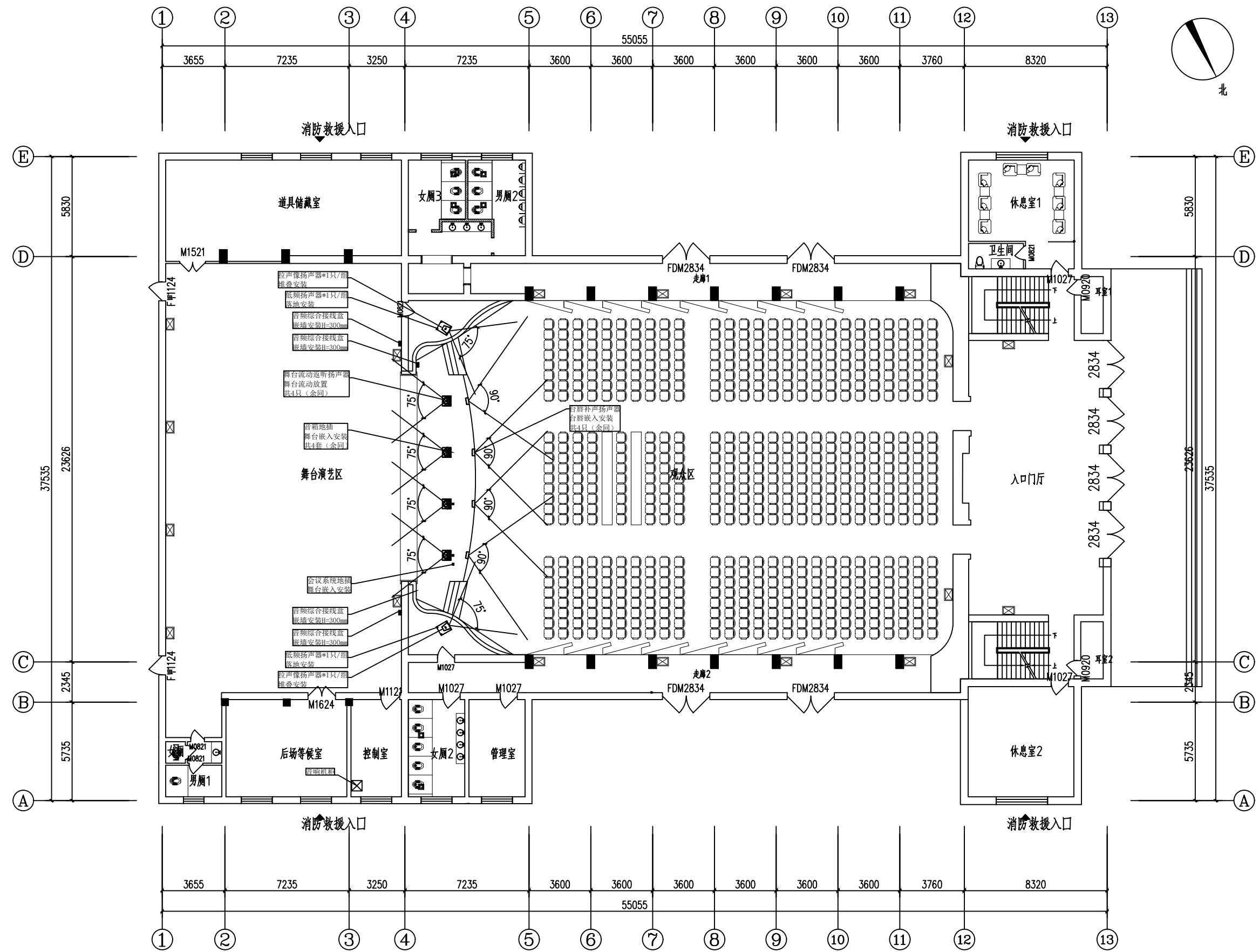
一层平面布置图
